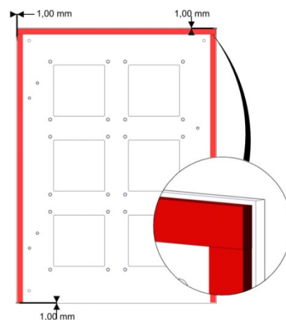
Abb. 2: Montage Frontlattendichtung
