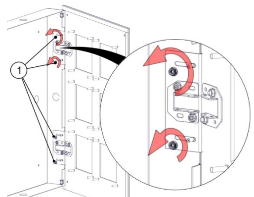
Abb. 1: Unterputzkasten montieren
