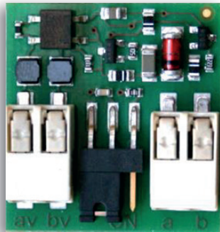
Video-2-Draht Filter-Platine FVW3040-0000
