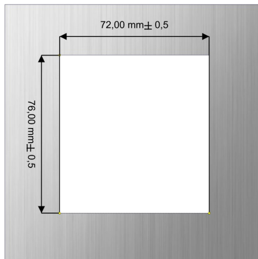
Abb. 1: Größe Frontplattenausschnitt
