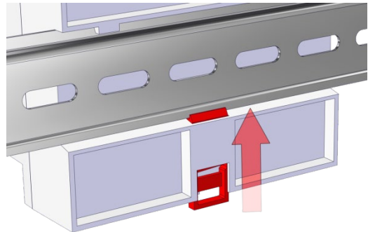
Abb. 3: Einrasten
