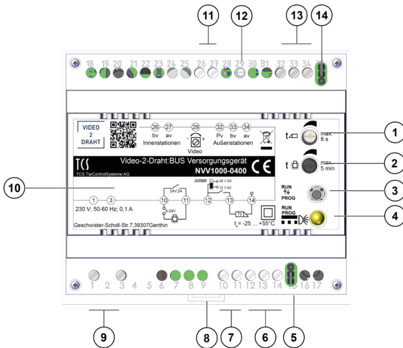
Abb. 1: Geräteübersicht NVV1000-0400
