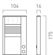
Video-Außenstation Serie AVC
