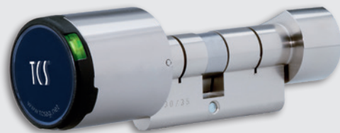
1x Schließzylinder (dreiteilig)
