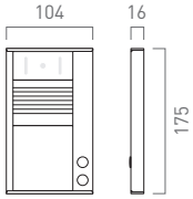
Video-2-Draht Außenstation Serie AVC
