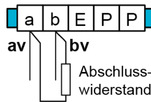
Abb. 1: Anschluss, Beispiel ISW5010
